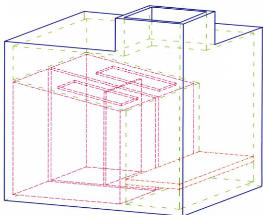
3D-Darstellung Erdmodul
