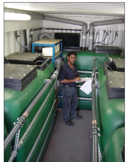
Kläranlage
