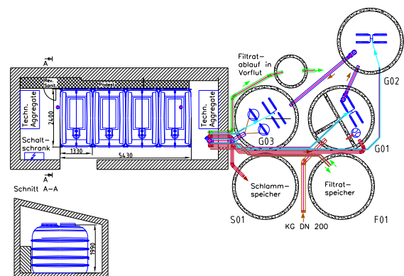
Aufstellplan BUSSE-MF
