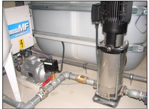
Brauchwasseraufbereitung mit Versorgungspumpe
