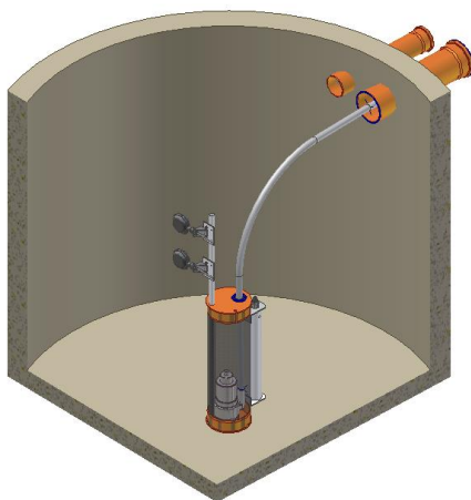
Grubenschema
