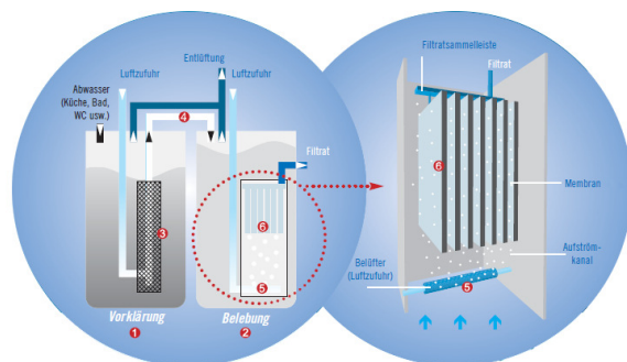
Verfahrensschema vollbiologische Membranfiltrationsanlage BUSSE-MF
