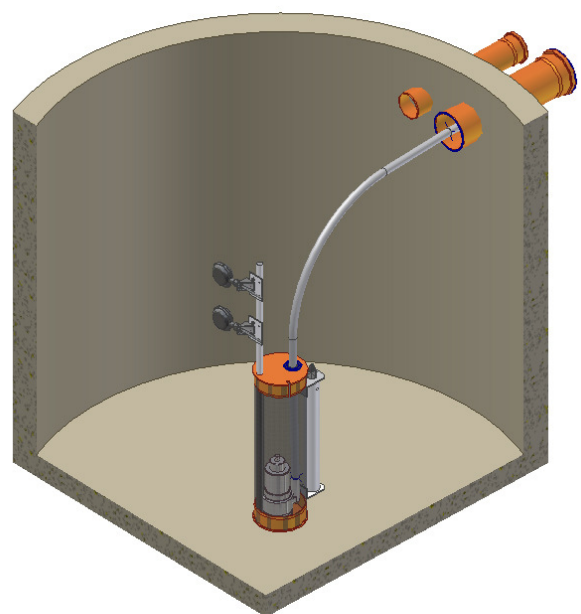
Abwassergrube mit Pumpeinheit ausgerüstet
