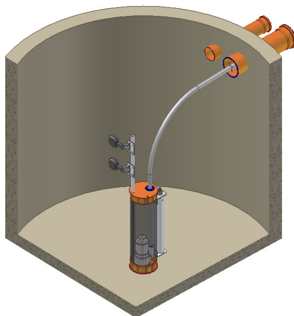
Abwassergrube mit Pumpeinheit
